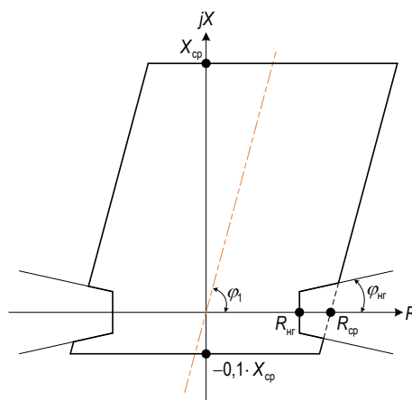
Рисунок 2.4 – Характеристика срабатывания отключающего РС ДФЗ
