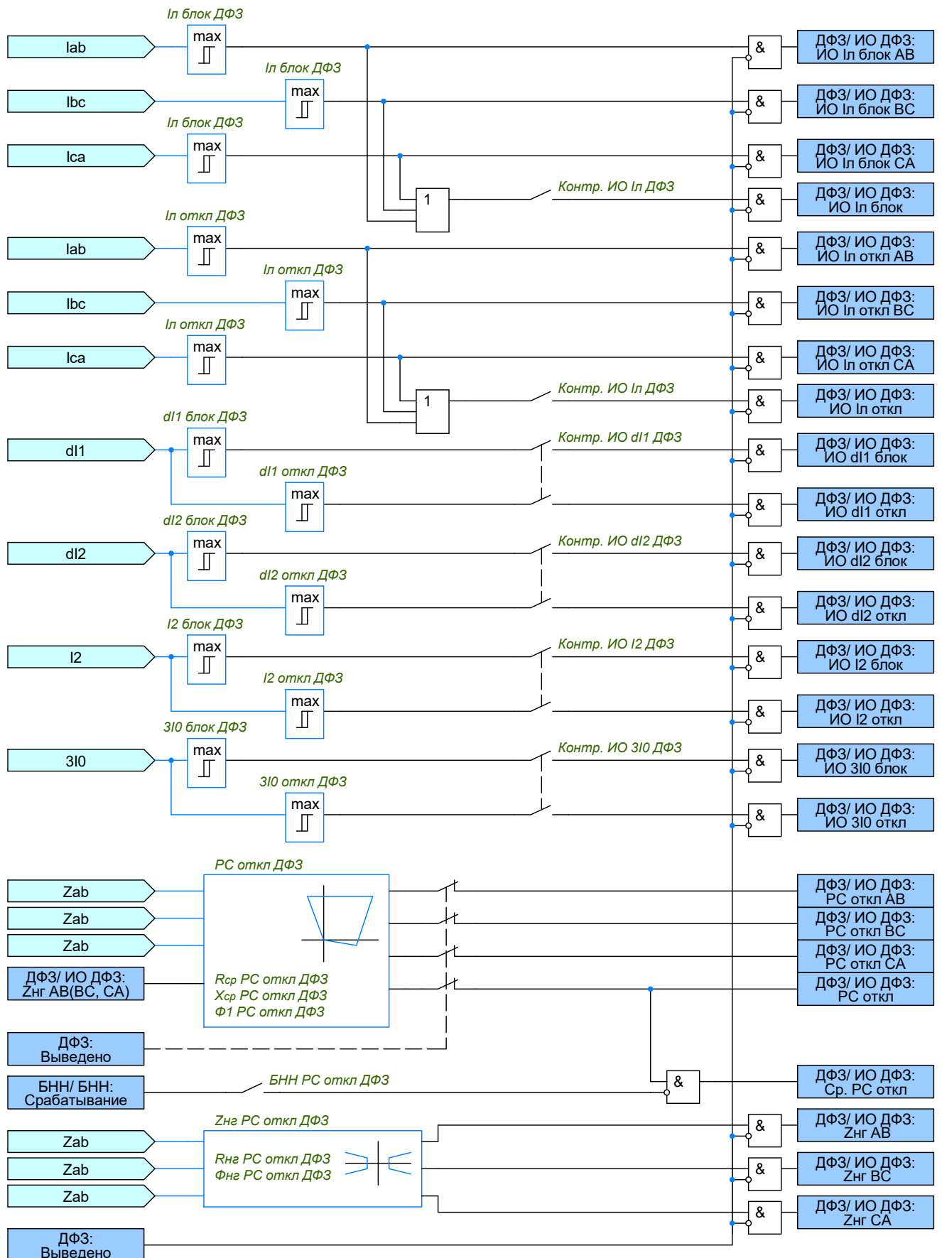
Рисунок 2.8 – Измерительные органы ДФЗ
