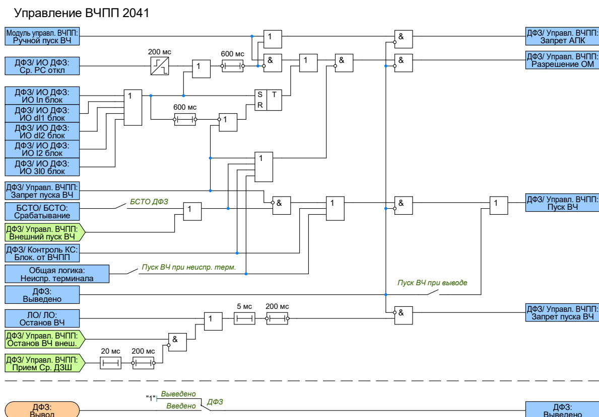
Рисунок 2.2 – Функциональная схема управления ВЧПП (ДФЗ)
