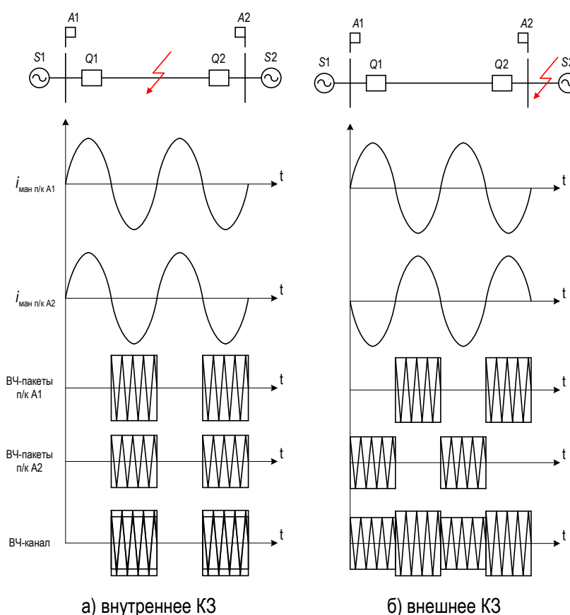
Рисунок 2.5 – Принцип действия ДФЗ
