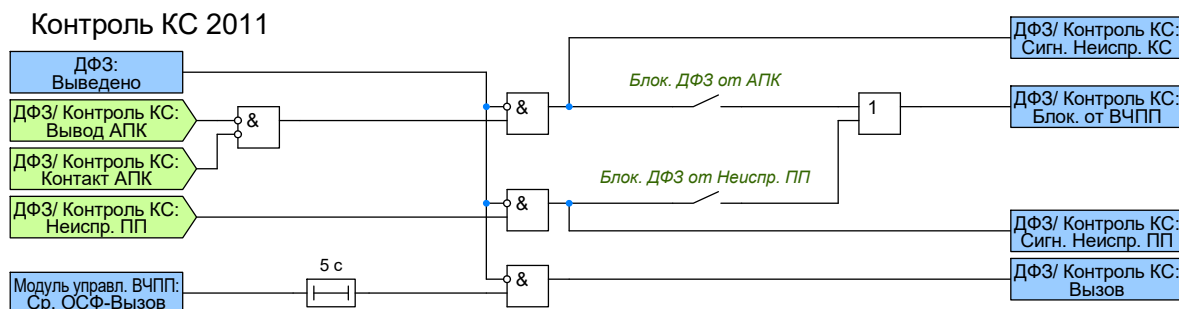
Рисунок 2.3 – Функциональная схема контроля ВЧ-канала связи
