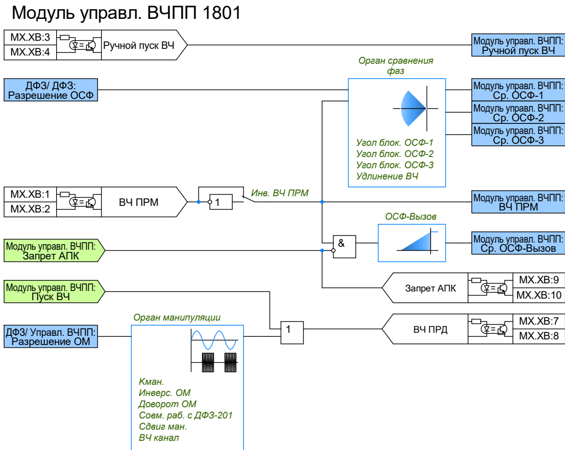
Рисунок 2.1 – Модуль управления ВЧПП
